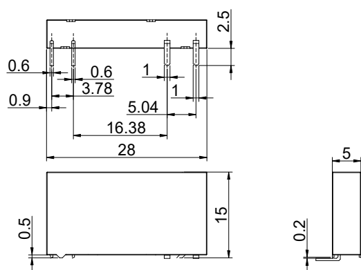
外形尺寸图
