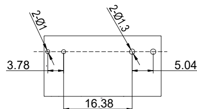
(底视图)
