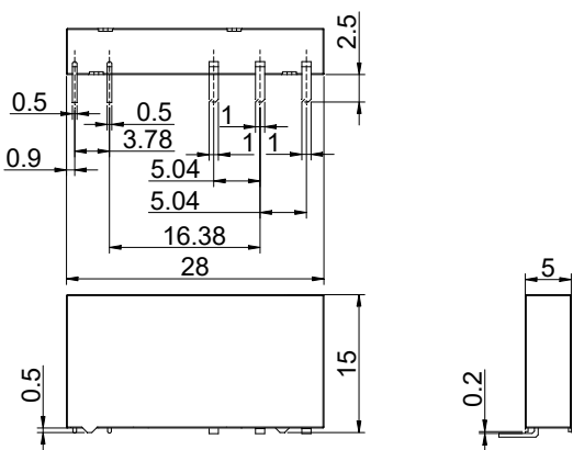
外形尺寸图
